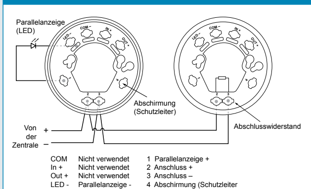
Anschlussplan Sav-Wire-Sockel
